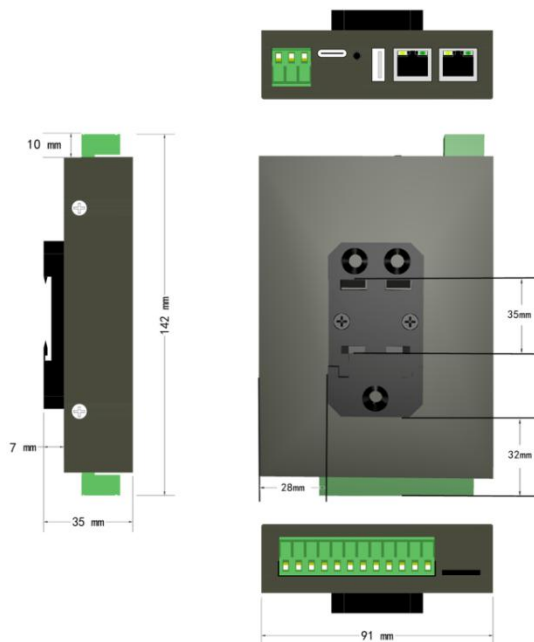
DIN Rail Mount
